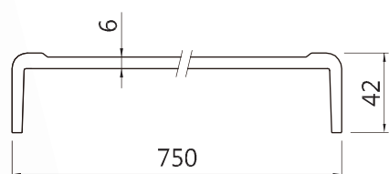
最大長度 2800 mm / SFB750 型
