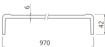
最大長度 2800 mm / SFB970 型
