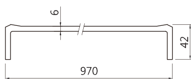
最大長度 2800 mm / YFB970 型
